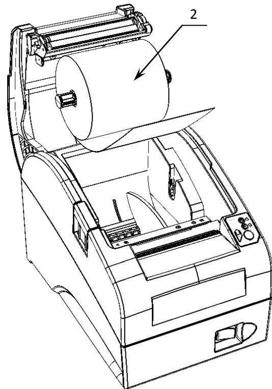
Рисунок 9. Установка ЧЛ
